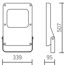
FL-Sport 170/210
